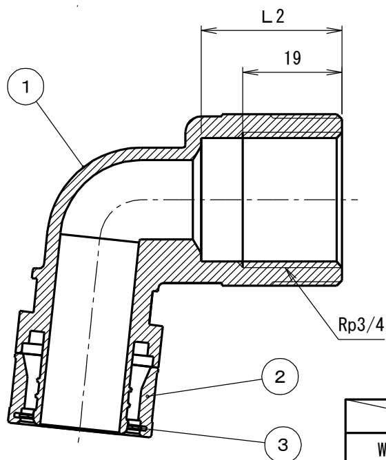
A-A断面図
